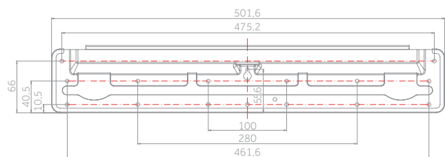
MONTAGEABMESSUNGEN
